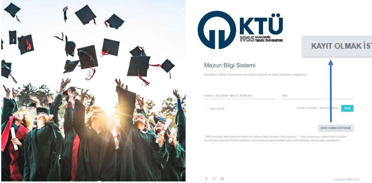
Şekil 1: Giriş Sayfası
